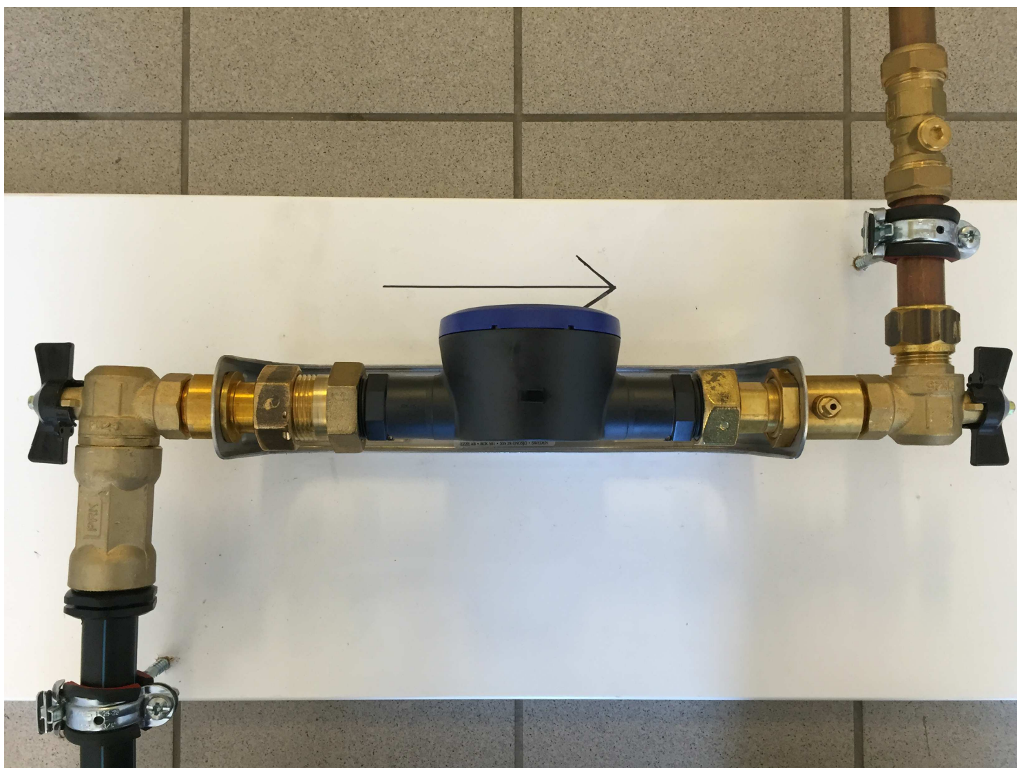
Exempel på mätarplats med återströmningskydd.
