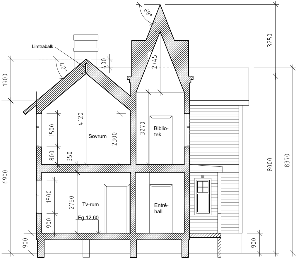
SEKTION A-A
