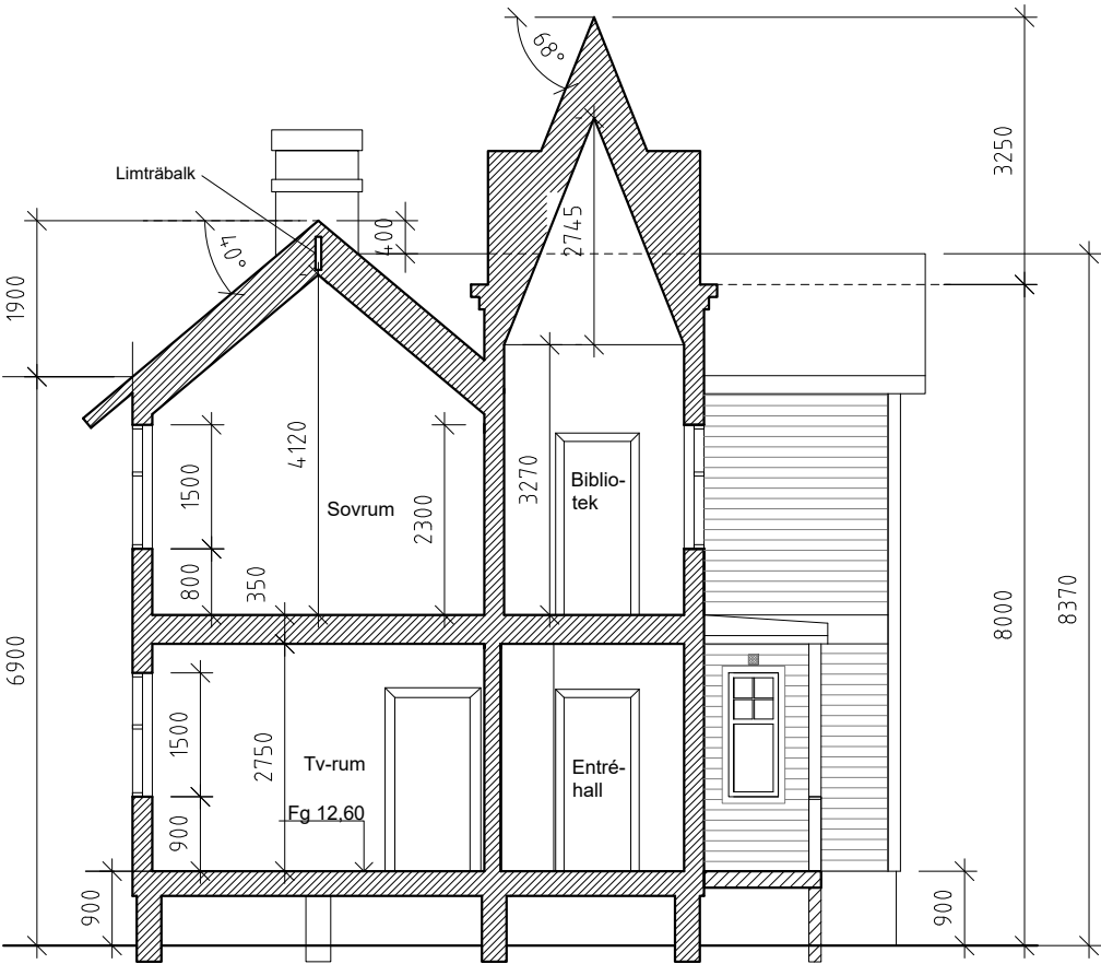
SEKTION A-A
