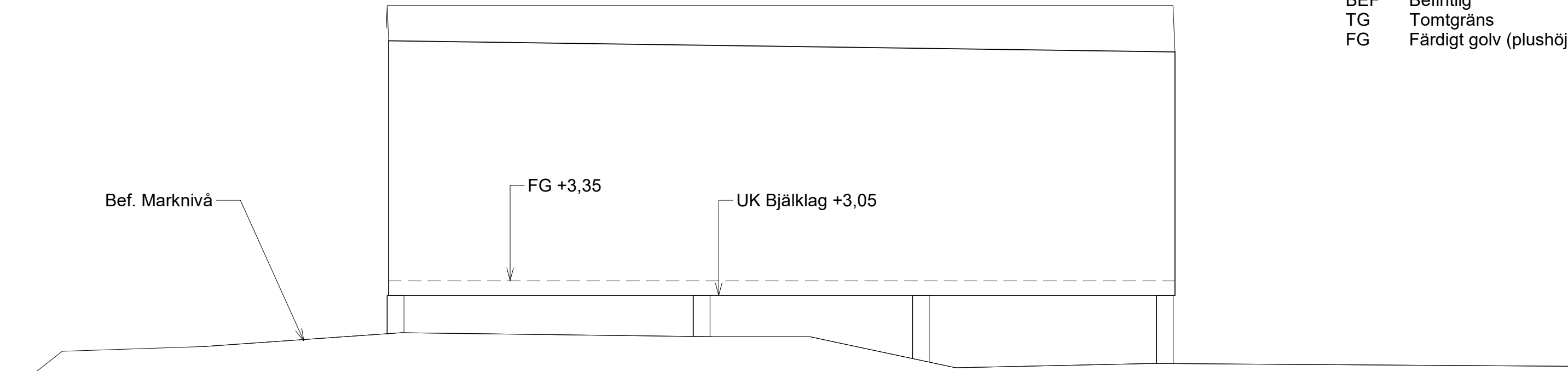
1 Ny Sektion 1-1 1 : 100
