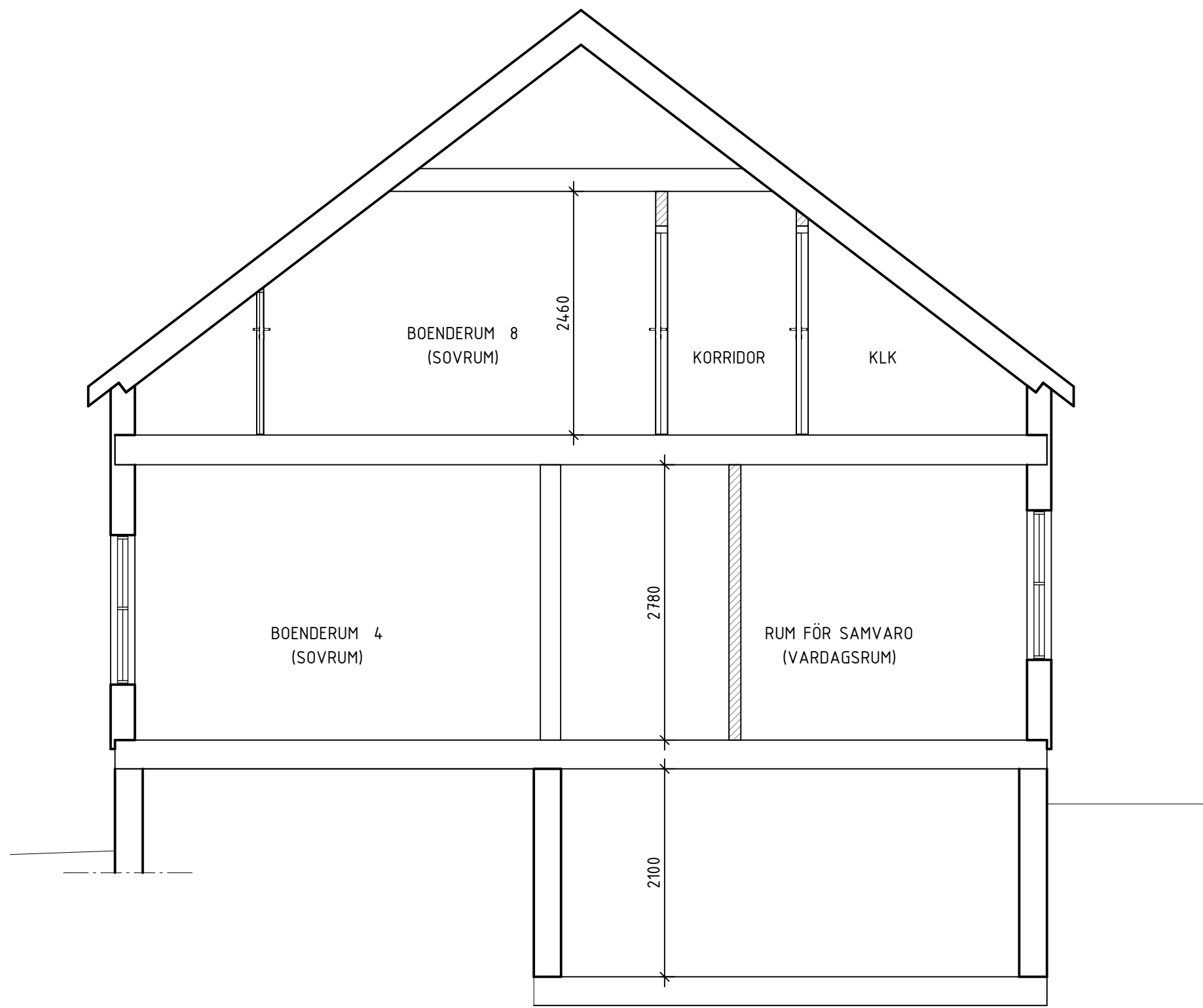
SEKTION A-A, HUVUDBYGGNAD
