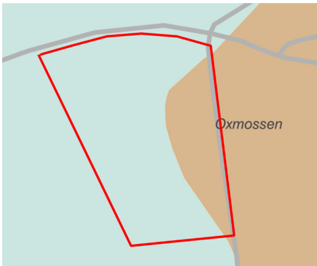
Utdrag ur SGU:s jordartskarta 2025 med planområdet markerat i rött.
