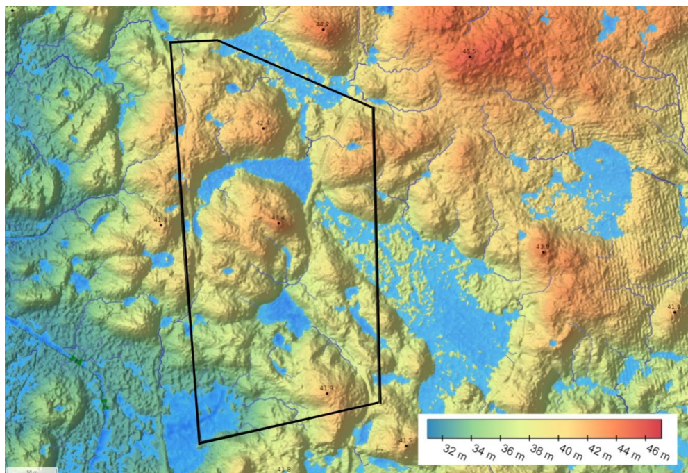
Terrängmodell (nationella höjddatabasen) samt uppskattning av ytliga avrinningsvägar och översvämmade ytor vid ett 22 mm regn. Planområdets ungefärliga läge illustreras med svart linje och avrinningsvägar samt stående vatten i blått (Scalco Live, 2022).
