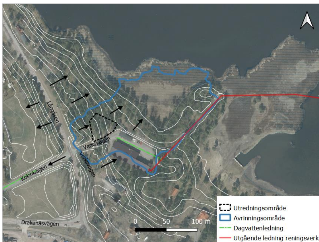
Figur 4. Avrinningsområde och planområdet. Svarta pilar = teoretisk strömningsriktning utifrån topografin
