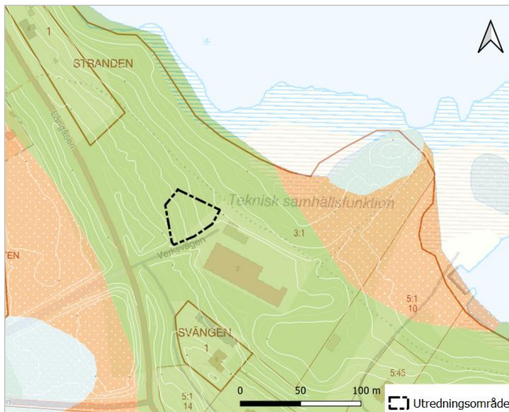
Figur 2. Jordartskarta från SGU och aktuellt utredningsområde. Grön area = isälvssediment
