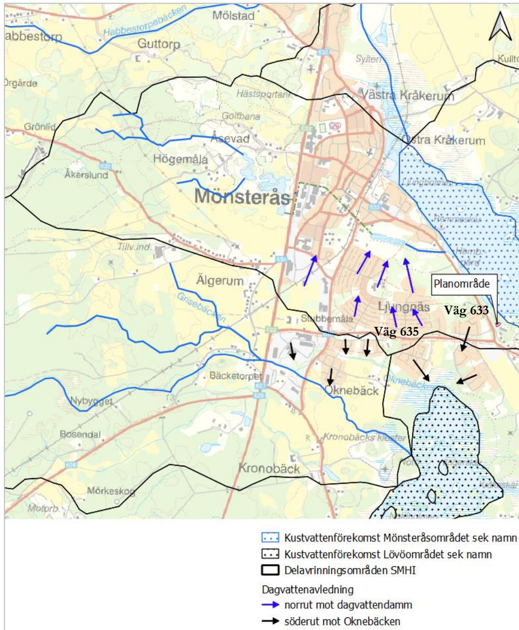
Figur 3. Översigtskarta med avrinningsområden, vattenförekomster och dagvattenavledning
